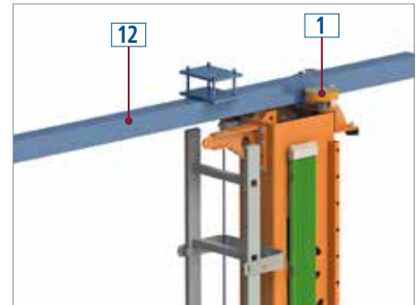
Châssis (1) et rail supérieur (12).
